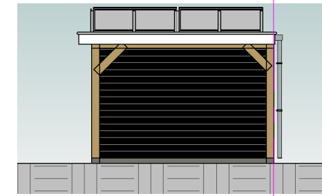
Rechtergevel
