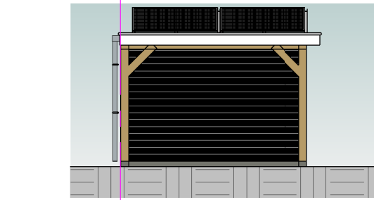
Linkergevel
